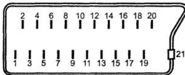
Рисунок В.1 - Расположение и нумерация контактов соединителя
